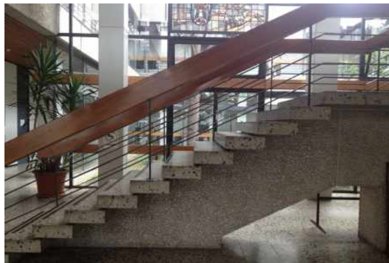
Holzbrüstung + Handläufe Treppen Bestand sichern / aufbereiten
